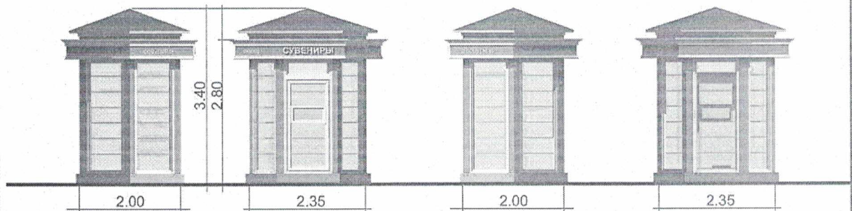
ТОРЦЕВОЙ ФАСАД
