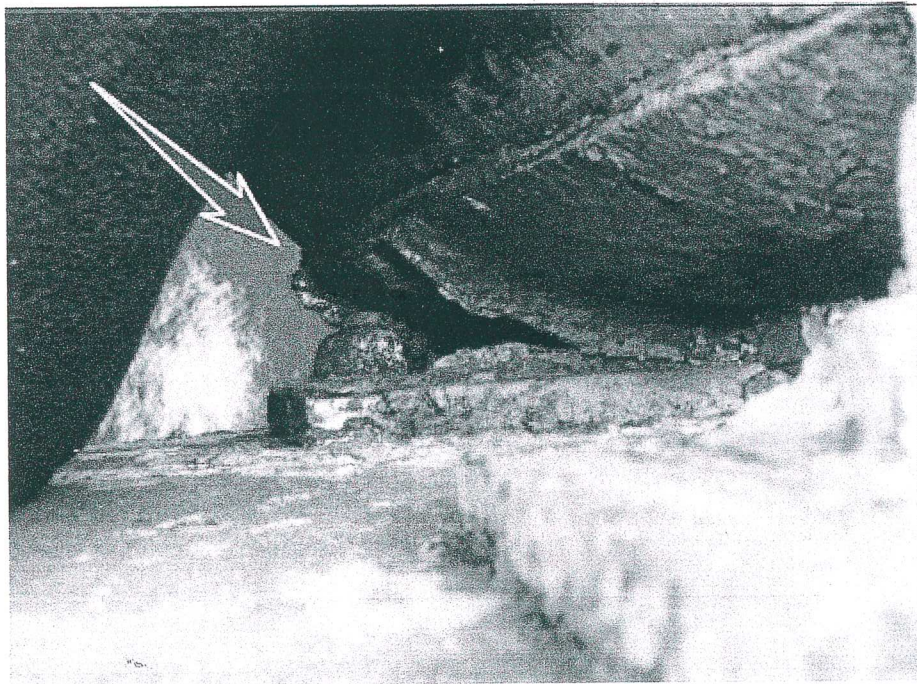
Рис. 3.4.4 Разрушение элементов крепления отбойных устройств
